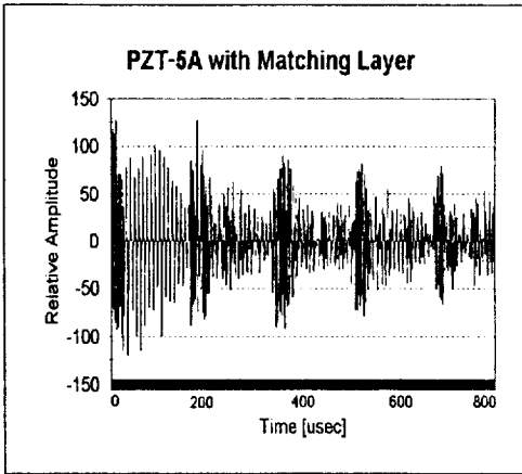
그림 8. 정합층을 가진 PZT-5A 탐촉자의 반사파 응답 Fig. 8. Pulse echo response of PZT-5A transducer with matching layer.
