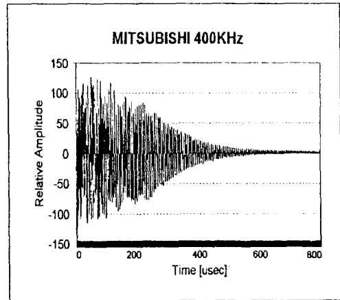
그림 7. 미쯔비시 탐촉자의 임펄스 응답 Fig. 7. Impulse response of MITSUBISHI Transducer
