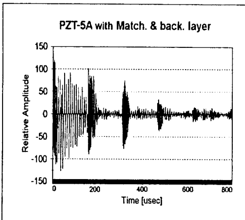
그림 9. 정합층과 후면층을 가진 PZT-5A 탐촉자의 반사파 응답. Fig. 9. Pulse echo response of PZT-5A transducer with matching and backing layers.
