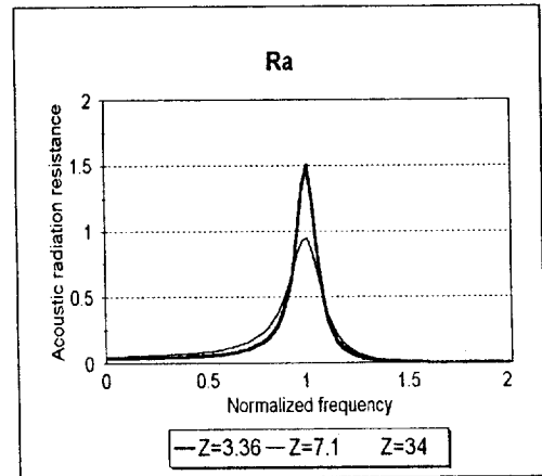
그림 3. 후면층이 있는 경우 정합층에 의한 음향방사저항의 변화
