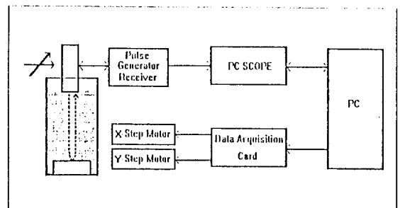
그림 11. 측정장치의 블럭도 Fig. 11. Block Diagram of measurement system.
