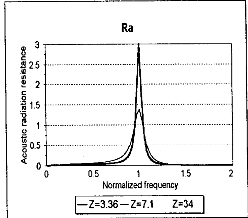
그림 2. 후면층이 없는 경우 정합층에 의한 음향방사저항의 변화
