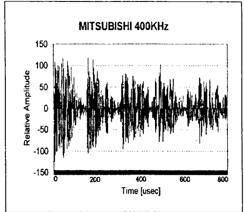
그림 10. 미쓰비시사 탐촉자 5의 반사파 응답 Fig. 10. Pulse echo response of MITSUBISHI transducer.
