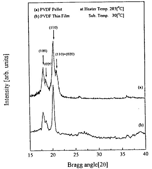
그림 4. PVDF 유기박막의 X선 회절패턴
