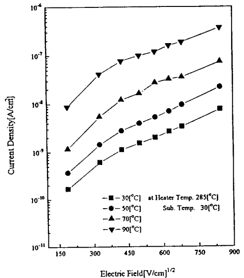
그림 9. PVDF 유기박막의 온도 변화에 따른 쇼트키 특성
