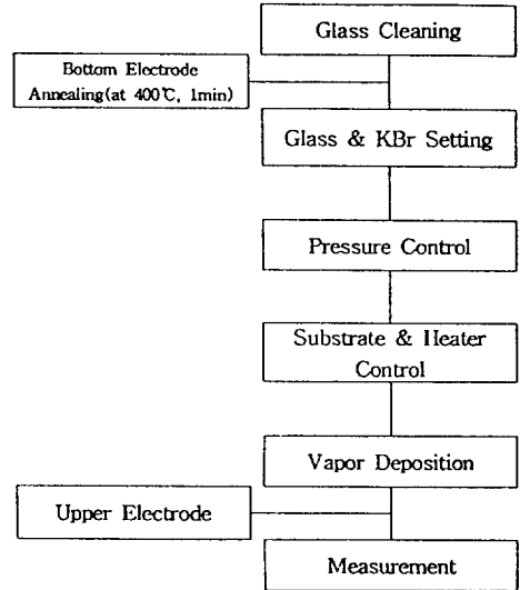
그림 2. PVDF 유기박막의 제조 공정도
