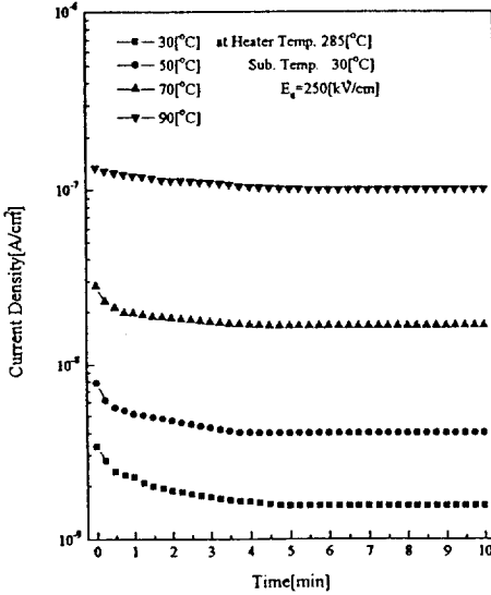
그림 6 . 온도에 따른 PVDF 유기박막의 시간 대 전류밀도특성
