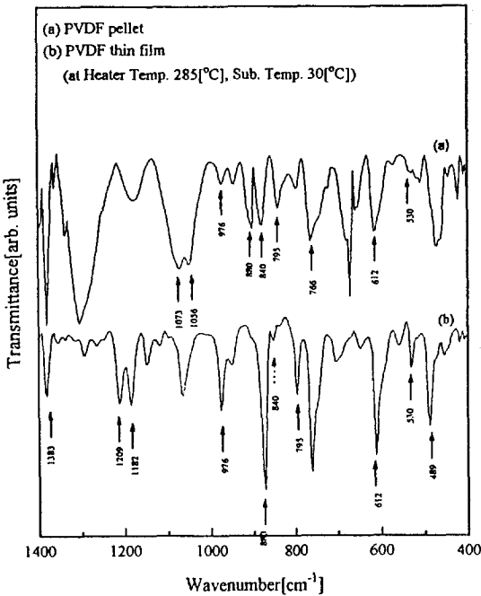
그림 5. PVDF 유기박막의 적외선흡수분광스펙트라
