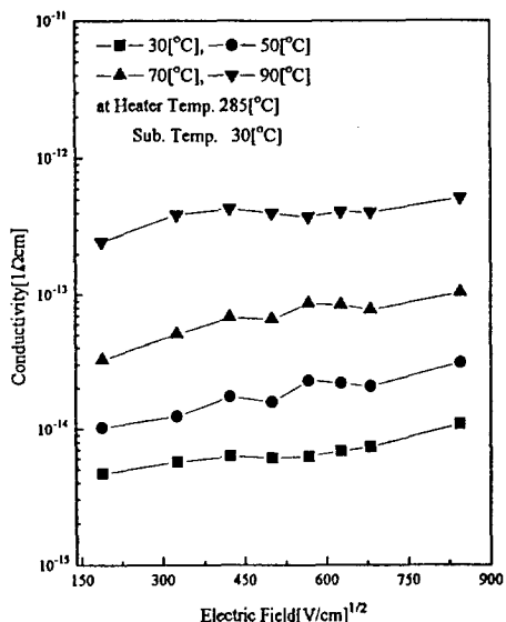
그림 10. PVDF 유기박막의 온도 변화에 따른 풀-프렌켈 전도 특성
