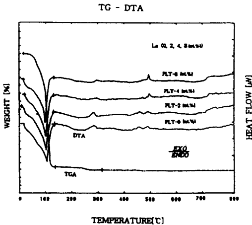
그림 2. La첨가량에 따른 PLT sol의 DT/TGA곡선.
