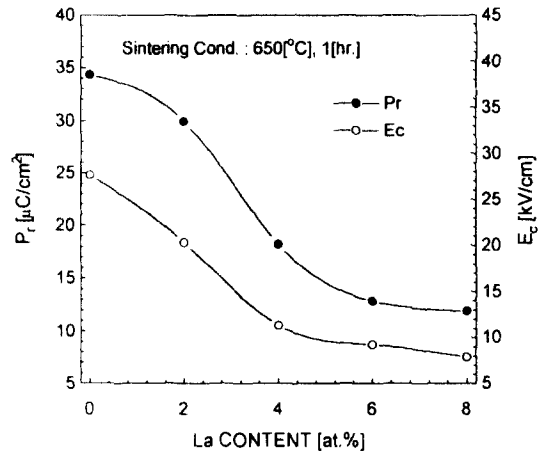
그림 6. La첨가량에 따른 PLT박막의 잔류분극 및 항전계
