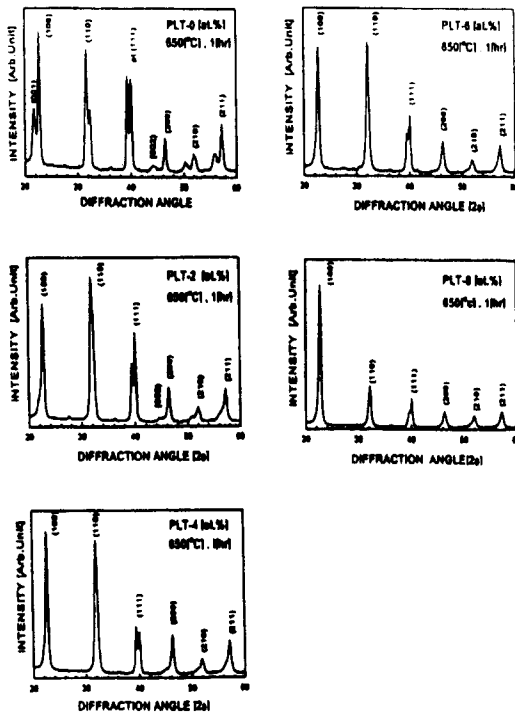
그림 3. La첨가량에 따른 PLT박막의 X-선 회절 모양.
