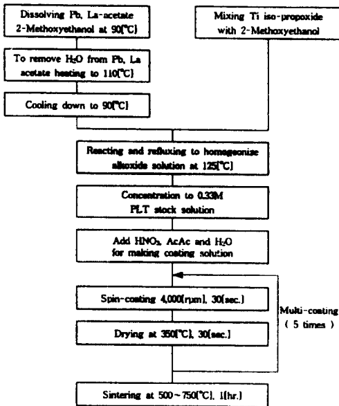
그림 1. PLT 박막의 제조과정
