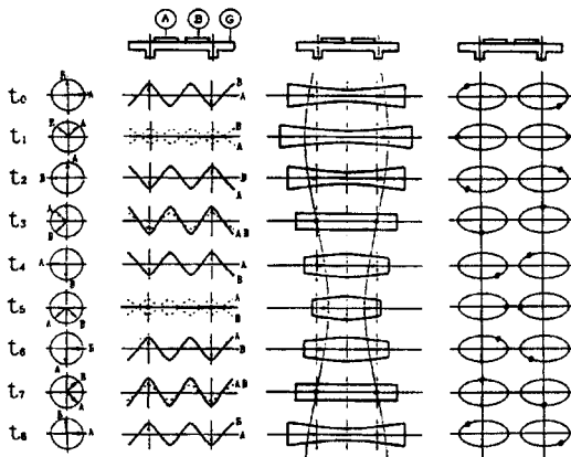
그림 1. 평판형 선형 초음파 모터의 동작원리
