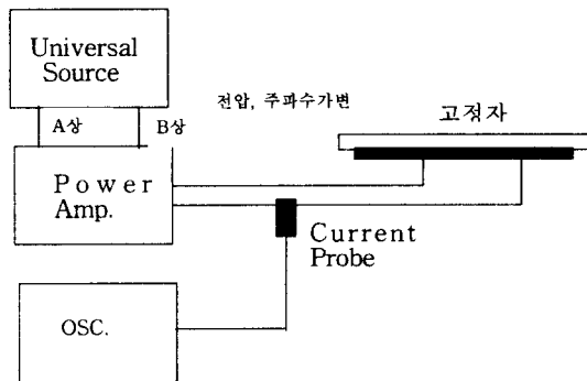
그림 3. 평판형 선형 초음파 모터의 구동 블록도 Fig. 3. Block diagram for driving plate-type linear ultrasonic motor
