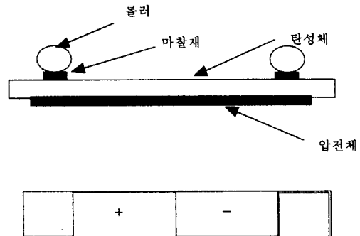
그림 2. 고정자의 구성도
