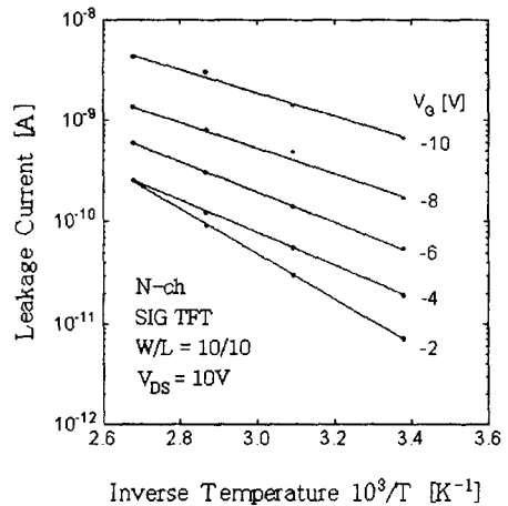
그림 5. Standard inverted gate 구조의 TFT에서 여러 가지 gate 전압에 따른 누설전류의 Arrhenius plot
