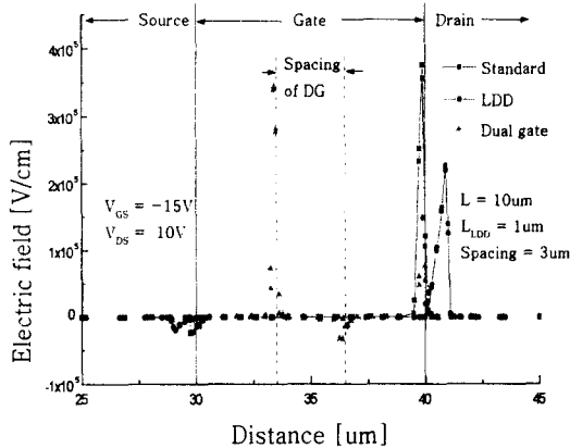
그림 7. 3 가지구조의 박막트랜지스터에 대한 채널 위치에 따른 전기장의 세기
