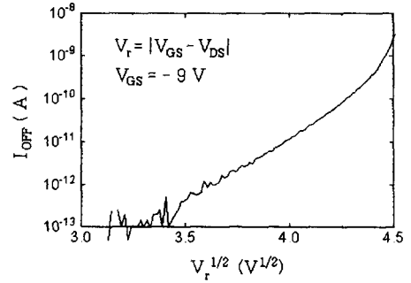
그림 4. SIG구조를 갖는 TFT의 역방향 드레인 전압 V_r 에 따른 누설전류( I_{OFF} )의 변화
