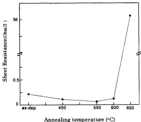
그림 6. 열처리 온도에 따른 Cu/TaN/Si 구조의 면저항 의존성.
