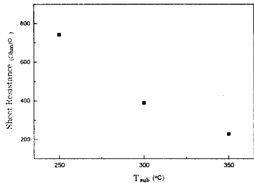
그림 1. 증착 온도에 따른 TaN 박막의 면저항 의존성.
