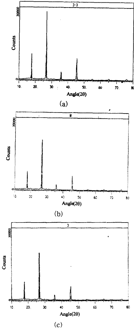
그림 2. 건전 시편과 열화시편(수소중과 공기중)의 X-ray 비교분석
