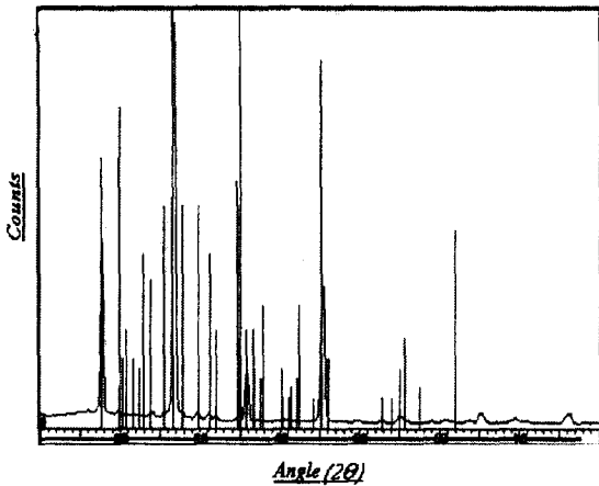
그림 4. X-ray 결과와 표준값의 비교(muscovite 7-32, KAl_2(OH)_2Si_3AlO_{10} ) Fig. 4. The comparison of X-ray results and standard data
