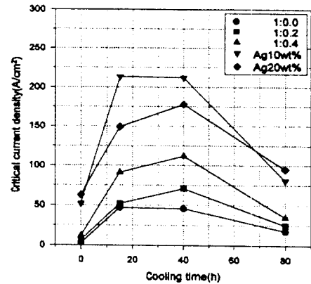
그림 5. 서냉시간에 따른 임계전류밀도
