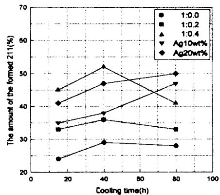
그림 6. Ag, \text{Y}_2\text{BaCuO}_5 첨가량을 달리한 시편의 서냉시간에 따라 형성된 \text{Y}_2\text{BaCuO}_5 상의 체적비
