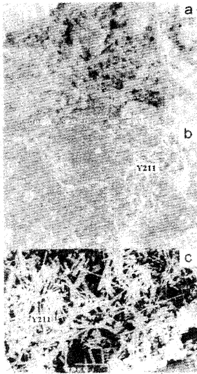
그림 4. 40시간의 서냉시간시 초전도벌크 파단면의 주사전자현미경사진
