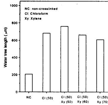
그림 9. (c) XLPE3의 추출 후 수트리 길이
