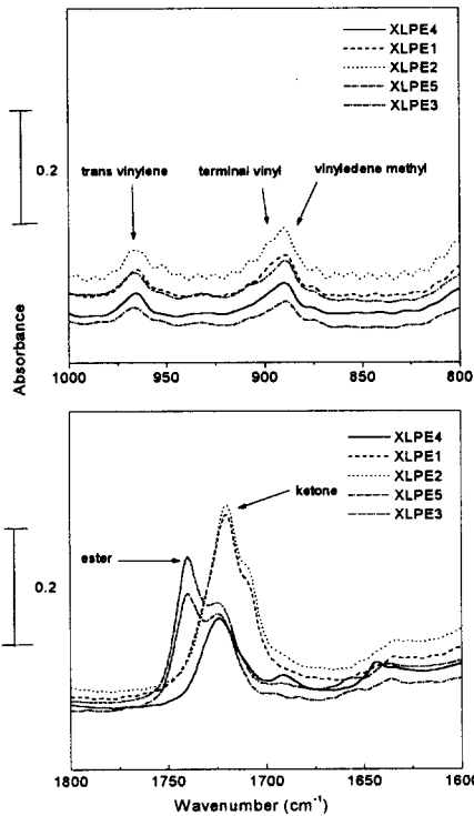
그림 2. (b) 가교 후 FTIR 스펙트럼 Fig. 2. (a) FTIR spectrum of crosslinked XLPEs
