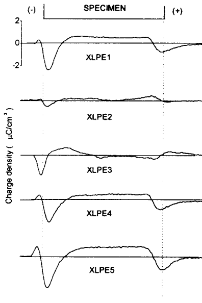
그림 10. (b) \text{CHCl}_3 50 °C & Xylene 50 °C 추출 후 전하분포 특성 Fig. 10. (b) Charge distributions after extraction ( \text{CHCl}_3 50 °C & Xylene 50 °C)
