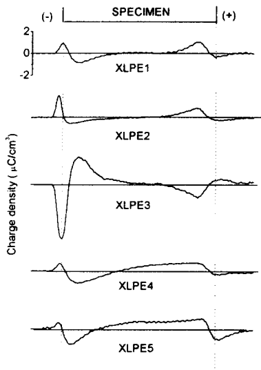
그림 10. (a) \text{CHCl}_3 50 °C 추출 후 전하분포 특성 Fig. 10. (a) Charge distributions after extraction ( \text{CHCl}_3 50 °C)
