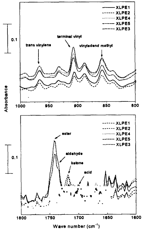
그림 2. (a) 가교 전 FTIR 스펙트럼 Fig. 2. (a) FTIR spectrum of uncrosslinked XLPEs
