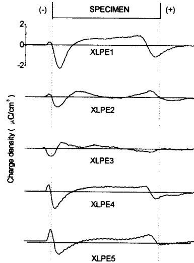
그림 10. (d) \text{CHCl}_3 50 °C & Xylene 70 °C 추출 후 전하분포 특성 Fig. 10. (d) Charge distributions after extraction ( \text{CHCl}_3 50 °C & Xylene 70 °C)
