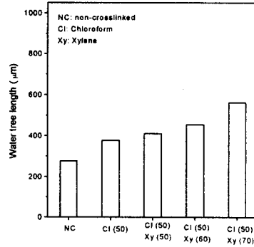
그림 9. (d) XLPE4의 추출 후 수트리 길이
