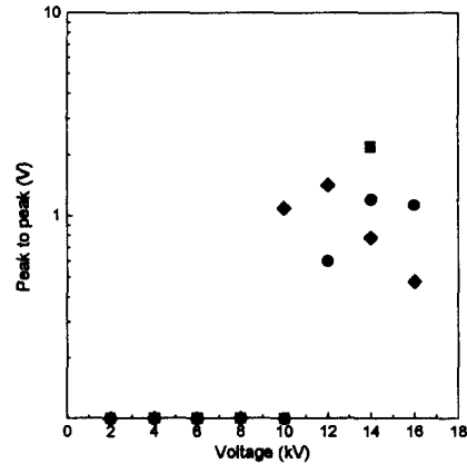
그림 7. XLPE1(●), XLPE2(◆), XLPE5(■)의 V_{pp} Fig. 7. V_{pp} of XLPE1(●), XLPE2(◆) and XLPE5(■)
