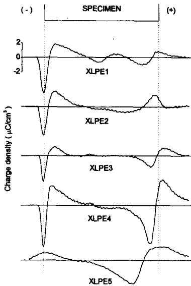
그림 4. 가교 후 전하분포 특성 (40 kV/mm) Fig. 4. Charge distributions of crosslinked XLPEs (40 kV/mm)
