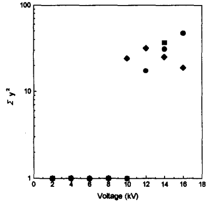
그림 6. XLPE1(●), XLPE2(◆), XLPE5(■)의 \Sigma y^2 Fig. 6. \Sigma y^2 of XLPE1(●), XLPE2(◆) and XLPE5(■)
