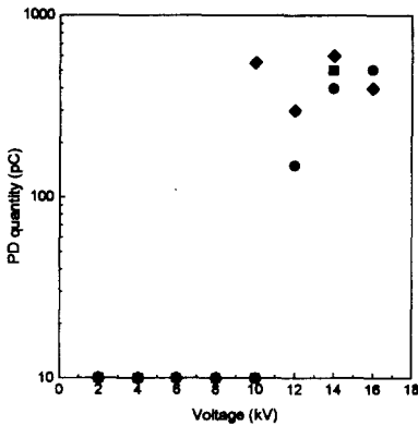
그림 5. XLPE1(●), XLPE2(◆), XLPE5(■)의 부분방전량 Fig. 5. PD quantity of XLPE1(●), XLPE2(◆) and XLPE5(■)
