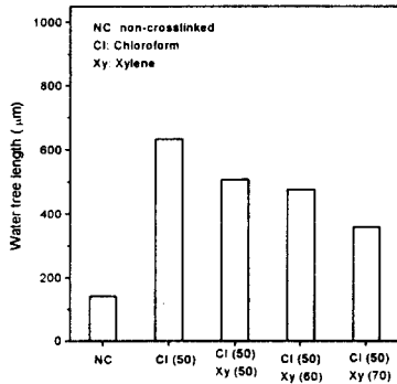
그림 9. (a) XLPE1의 추출 후 수트리 길이
