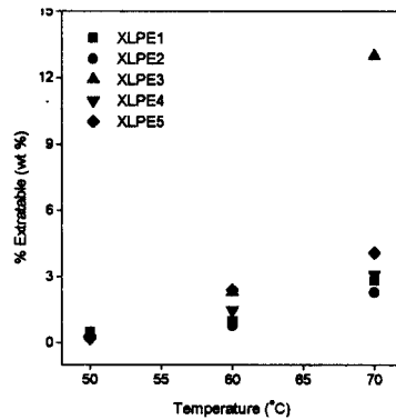
그림 8. 추출 온도에 따른 추출 양
