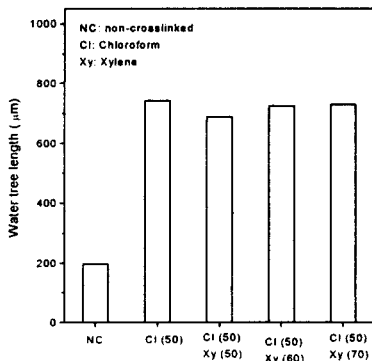
그림 9. (b) XLPE2의 추출 후 수트리 길이
