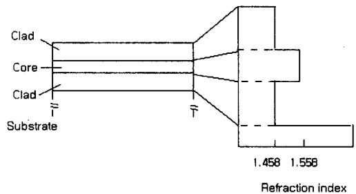
그림 10. 제작된 기판과 막의 굴절률 분포 Fig. 10. Refractive index profiles of the fabricated thin film and substrate
