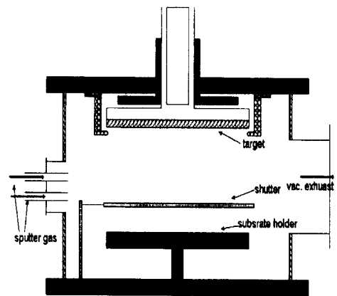
그림 3. 반응성 스퍼터링의 구조도
