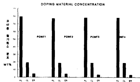
그림 6. 코어층내의 에르븀의 분포(불순물인 Al에 대한 첨가물들의 양을 질량비로 나타낸 것)
