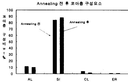
그림 7. 열처리 전후의 불순물첨가 결과 비교 Fig. 7. Doping material at corea after Annealing
