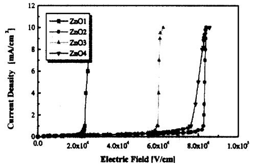
그림6 ZnO 바리스터의 전압-전류 특성 Fig. 6 The characteristics of voltage-current to ZnO varistors
