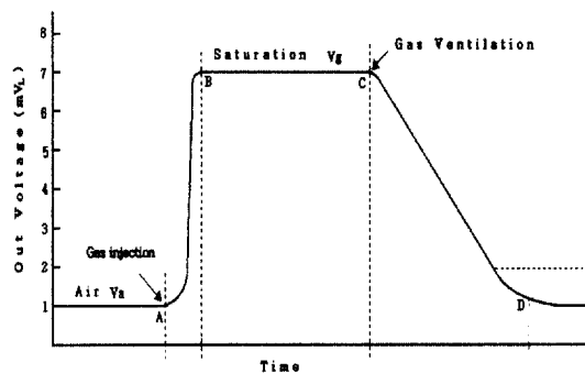
그림 3 센서의 출력특성
