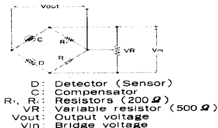
그림 2 휘스톤 브릿지
