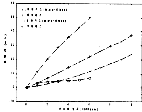
그림 9 인가전압 2.3 V에서의 센서출력특성 Fig. 9 Output characteristics of sensor at 2.3
