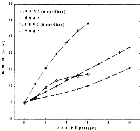
그림 7 인가전압 2.1 V에서의 센서출력특성 Fig. 7 Output characteristics of sensor at 2.1 V
