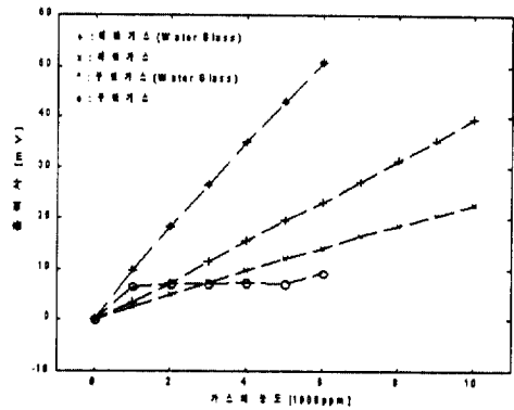
그림 8 인가전압 2.2 V에서의 센서출력특성 Fig. 8 Output characteristics of sensor at 2.2 V
