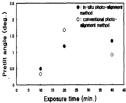
그림 3 폴리이미드 표면에 편광된 UV 광을 20분간 30° 경사 조사시의 조사시간에 따른 네마틱 액정의 프리틸트 각의 발생
