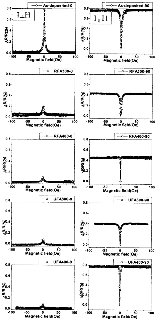
그림 5 증착후 1시간동안 자장열처리한 Ni_{81}Fe_{19} 박막의 열처리 온도와 방법에 따른 자기 저항곡선
