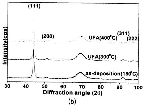
그림 2 열처리온도에 따른 Ni_{81}Fe_{19} 박막의 XRD 회절 패턴
