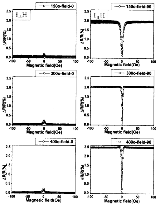
그림 9 자장내에서 증착된 Ni 81 Fe 19 박막의 증착온도에 따른 MR 곡선
