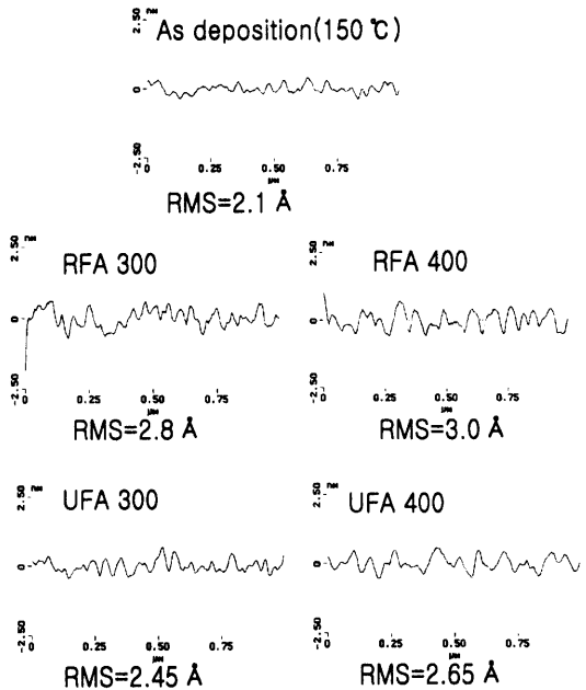
그림 4 증착후의 1시간동안 자장 열처리한 Ni 81 Fe 19 박막의 열처리 온도와 방법에 따른 단면그림 Fig. 4 Line profiles of the surfaces of Ni 81 Fe 19 thin films for 1hr ex-situ field annealing as a function of annealing temperature and annealing method.
