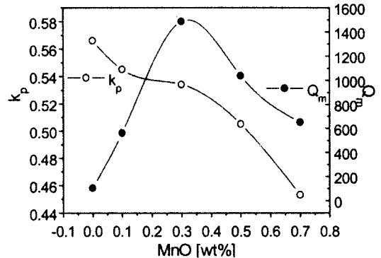
그림 8 MnO 첨가량에 따른 전기기계결합계수 k_p 와 기계적 품질계수 Q_m Fig. 8 Electromechanical coupling factor k_p and mechanical quality factor Q_m with the addition amount of MnO
