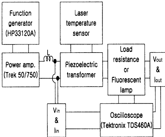
그림 2. 압전 트랜스포머의 구동 및 측정 시스템 Fig. 2. Driving and measuring system for piezoelectric transformer.
