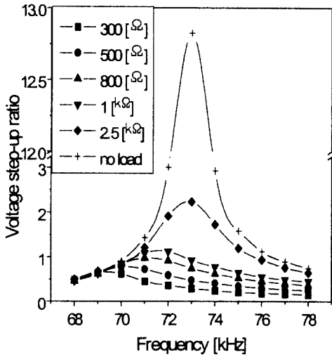
그림 9 주파수와 부하저항에 따른 승압비 Fig. 9 Voltage step-up ratio with frequency and load resistance
