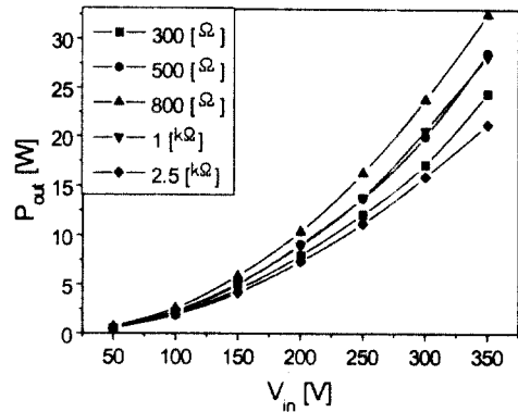
그림 11 입력전압에 따른 출력전력 Fig. 11 Output power with input voltage
