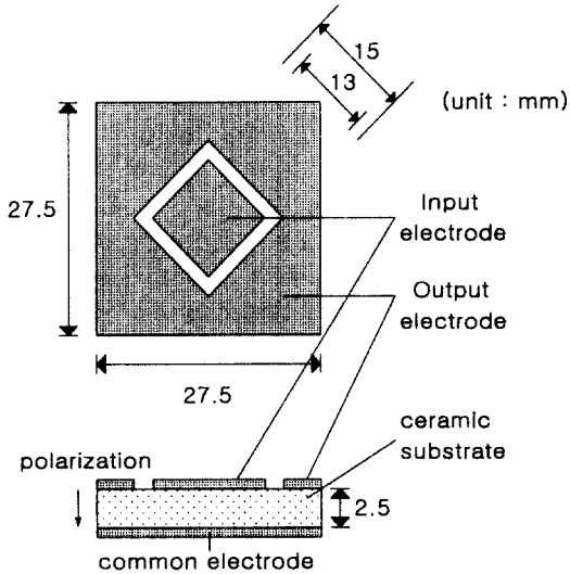
그림 1. 새로운 Diamond dot-Ring형 압전 트랜스포머의 구조
