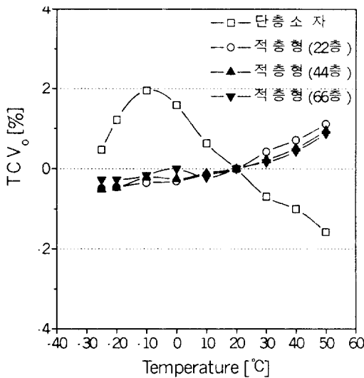
그림 8. 온도에 따른 출력전압의 온도계수 TCV_0 Fig. 8. Temperature coefficient of output voltage TCV_0 according to the temperature.
