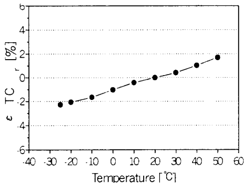
그림 5. 온도에 따른 유전율의 온도계수 TCε r Fig. 5. Temperature coefficient of dielectric constant( TCε r ) with temperature.
