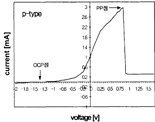
그림 3. 전기화학적 식각정지시 p-형 Si의 I-V 특성 곡선.
