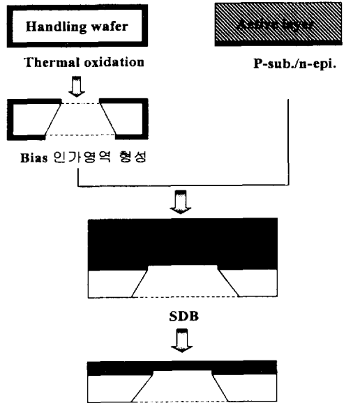
전기화학적 식각정지법에 의한 SDB SOI의 박막화
