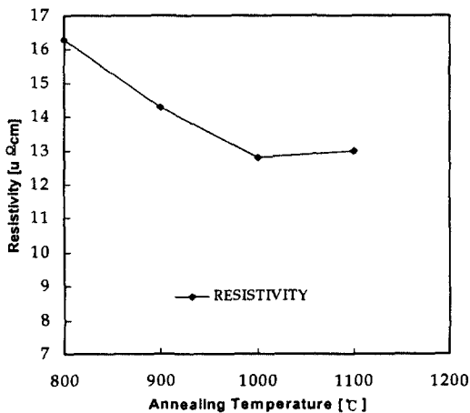
그림 2. MgO 박막위에 증착된 백금박막의 열처리 온도에 따른 비저항값의 변화(열처리 시간 : 120분).
