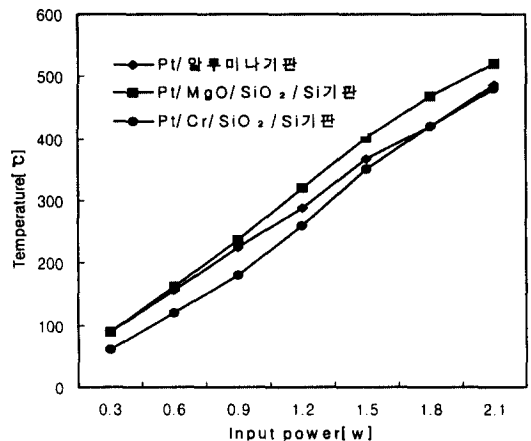
그림 7. 기판 및 매개층에 따른 백금박막형 미세발열체의 발열특성. Fig. 7. Thermal characteristics of Pt thin-film type microheater according to substrate and medium layer, respectively.
