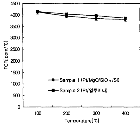
그림 6. Si 및 알루미늄기판 위에 각각 제작된 박막형 Pt-RTD의 온도에 따른 TCR값 변화. Fig. 6. Variations of TCR value of thin-film type Pt-RTD fabricated on Si and Al 2 O 3 substrates, respectively.
