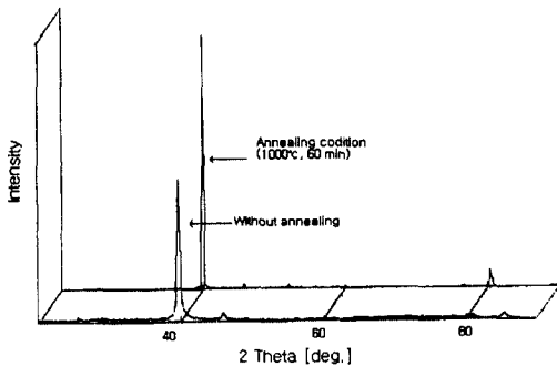
그림 5. Pt/MgO 이중박막의 열처리에 따른 XRD 회절패턴 분석. Fig. 5. XRD patterns of Pt/MgO bilayer thin-film according to annealing.
