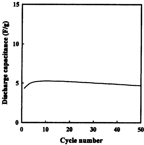
그림 2. PAn 전극의 1mA/cm 2 전류 밀도에서 방전 전기량.
