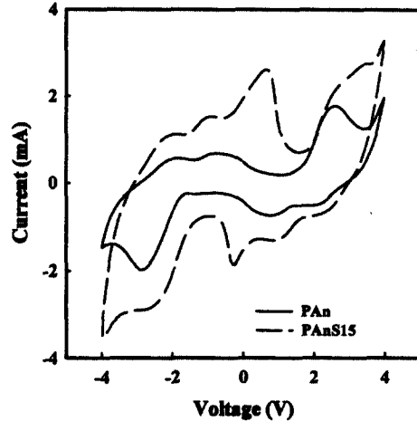
그림 1. PAn과 PAn composite 전극의 cyclic voltammogram.
