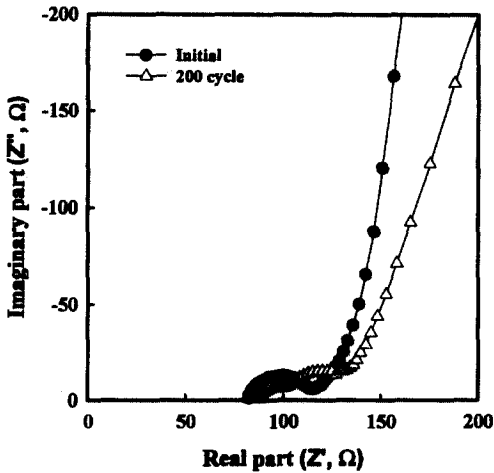
그림 5. 싸이클에 따른 PAn composite cell의 임피던스 스펙트럼.
