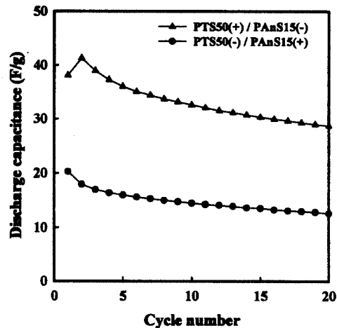
그림 10. PTS50/PAnS15로 구성된 supercapacitor cell의 방전 전기량.
