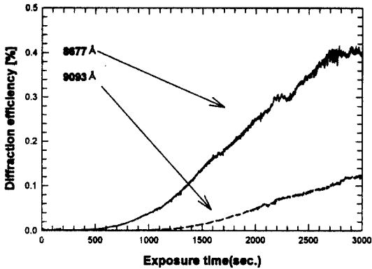
그림 5. As_{40}Ge_{10}Se_{15}S_{35} 박막의 두께 8677 Å과 9093 Å에 따른 회절효율.
