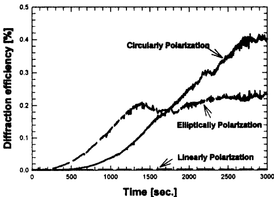
그림 4. 원형, 타원, 선형편광형태별 광유기 시간에 대한 회절효율.
