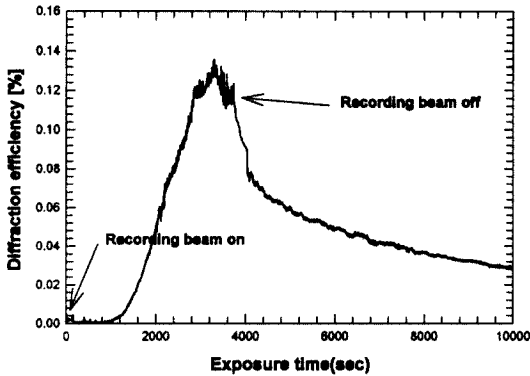
그림 3. 기록광파의 on-off시 원형편광(RCP)을 기록광파로 한 회절효율 변화.
