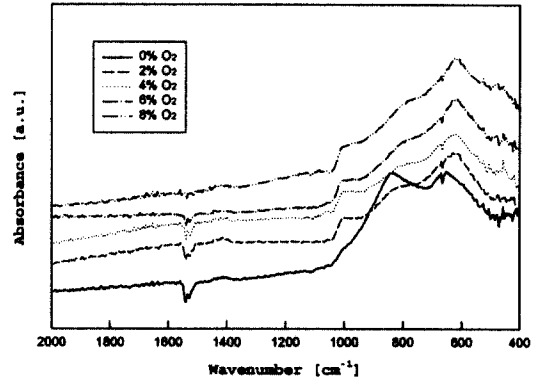
그림 4. 바나듐 산화막의 FTIR 스펙트럼.
