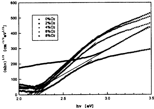
그림 7. 바나듐 산화막에 대한 입사광 에너지 h\nu 의 함수로서 (\alpha h\nu)^{1/2} 의 변화.
