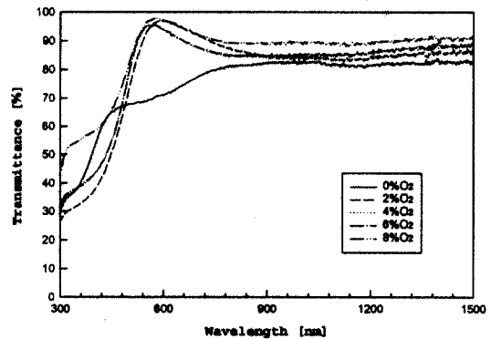
그림 5. 바나듐 산화막의 광투과 스펙트럼.
