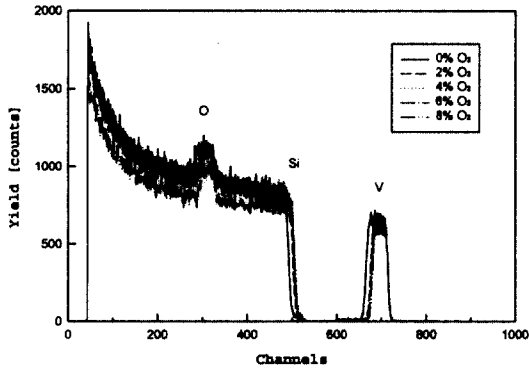
그림 3. 바나듐 산화막의 RBS 스펙트럼.
