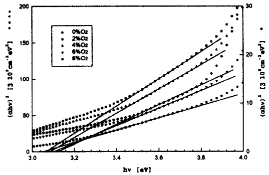
그림 8. 바나듐 산화막에 대한 입사광 에너지 h\nu 의 함수로서 (\alpha h\nu)^2 의 변화.
