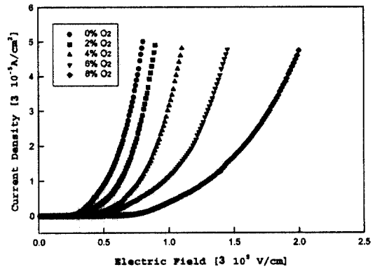
그림 9. 바나듐 산화막의 전류밀도-전계 특성.
