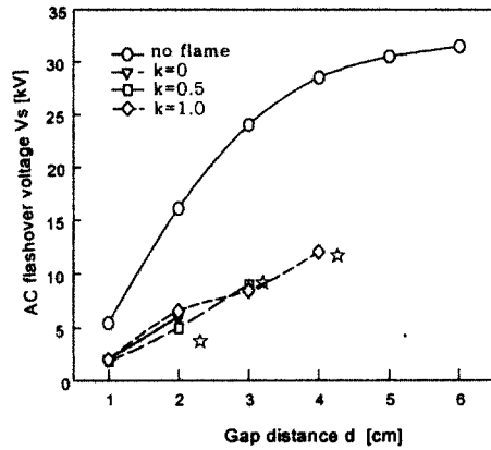
그림 5. 침대침갭에서 교류섬락전압과 갭간 거리의 관계.
