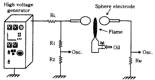
그림 1. 실험 장치의 개략도.
