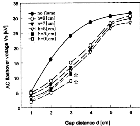
그림 7. 침대침갭에서 교류섬락전압과 갭간 거리의 관계.
