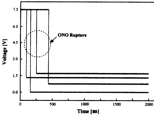
그림 6. 앤티퓨즈의 절연과괴 시간 (프로그램 전압 : 7.5 V).
