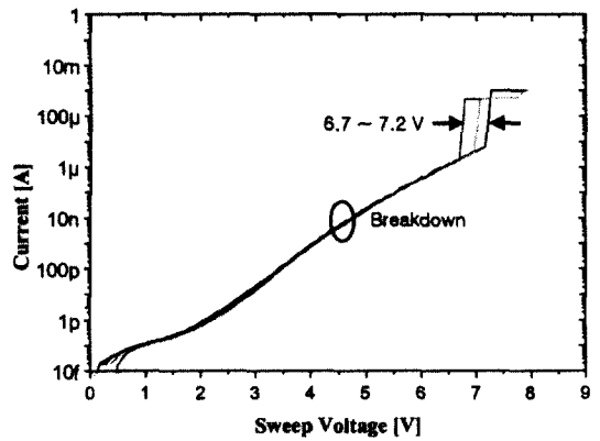
그림 5. 엔티퓨즈 프로그램의 I-V 특성. Fig. 5. I-V characteristics in programming antifuses.
