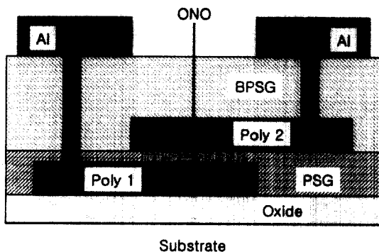
그림 1. 엔티퓨즈의 구조. Fig. 1. An antifuse structure.
