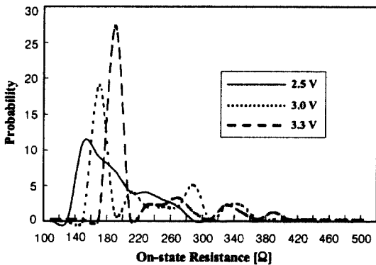
그림 7. 프로그램 후 저항 분포.
