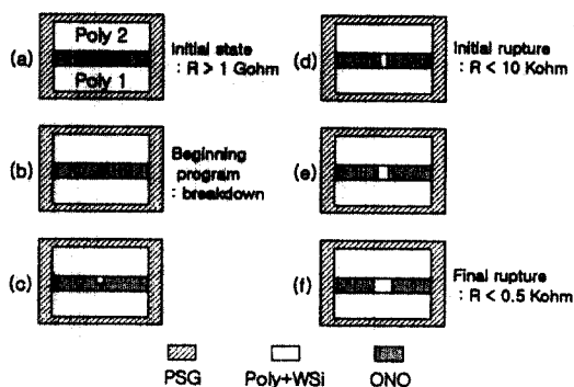
그림 3. 엔티퓨즈의 프로그램 진행 과정. Fig. 3. The progression of programming antifuse.
