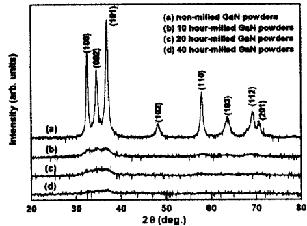
그림 1. 연마시간에 따른 GaN 분말의 X선 회절 패턴.
