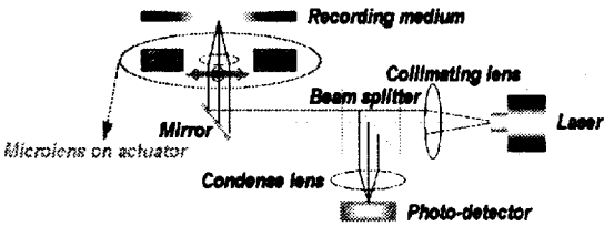
그림 7. 마이크로 렌즈의 위치제어를 통한 광기록 장치로의 응용 개념도. 마이크로 렌즈가 좌우로 움직이면 렌즈를 통과한 빛이 좌우로 위치를 변동하게 되어서 track-following이 가능하다.
