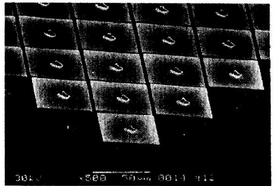
그림 13. 알루미늄 표면 마이크로머시닝 기술로 제작한 마이크로 미러 어레이. 마이크로 미러의 크기는 50 \mu m이다.
