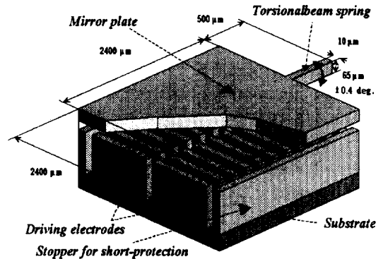
그림 9. 한 변의 크기가 2.4 mm인 미러를 구동시키는 시스템의 예. 미러는 단결정 실리콘이고 0.4 도 정도 회전이 가능하다.
