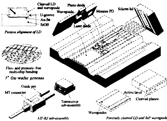
그림 1. 집적화된 광송수신 모듈(10)
