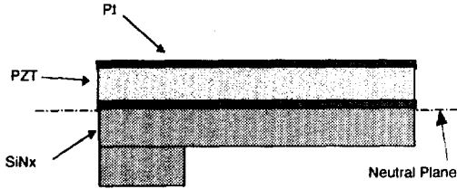
(b) 단면도
