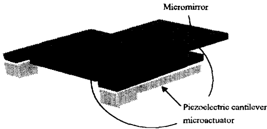
(a) 입체도
