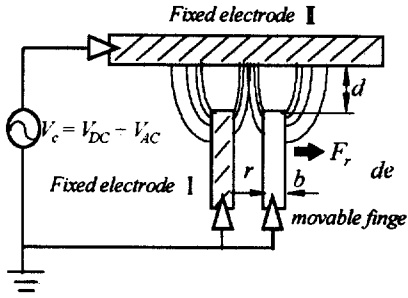
(a) 동작원리
