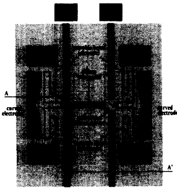
(a) 스위치 구조
