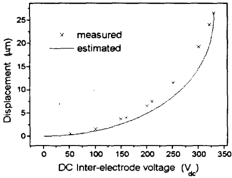
(b) 바이어스 전압에 따른 구동진폭 변화
