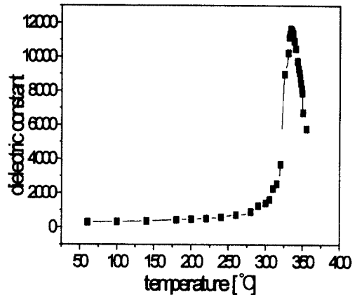
그림 3. Pb(La,Ce)TiO 3 세라믹스의 온도에 따른 유전상수.
