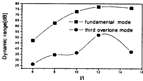
그림 2. 세라믹스 기판의 크기에 따른 1차, 3차 D.R(Dynamic Range).
