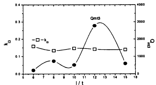
(b) 3차에서의 k_{b3} 및 Q_{m3}
