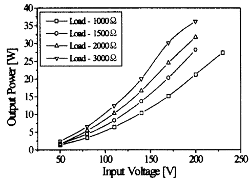
그림 9. 입력전압에 따른 출력전력. Fig. 9. Output power as a function of input voltage.
