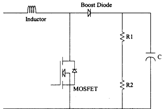
그림 5. 부스트 컨버터.
