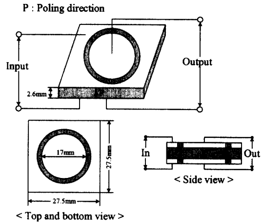
그림 1. 압전트랜스포머의 구조.
