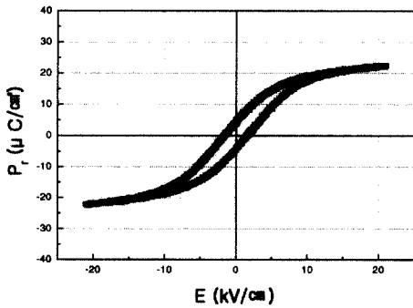
c) 20 layer stacking(10×10 mm 2 )
