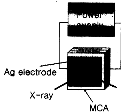
그림 1. 200 V로 인가된 적층형 세라믹 액츄에이터의 XRD 측정 모식도.
