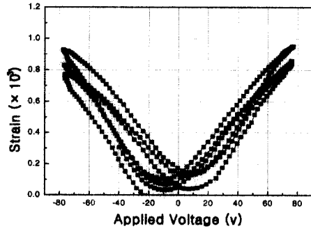
a) 10 layer stacking(5×5 mm 2 )
