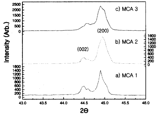
그림 6. 200 V의 전계가 인가된 적층형 세라믹 액추에이터의 X 선 회절 패턴 a) 10 layer stacking(5×5 mm 2 ) b) 10 layer stacking(10×10 mm 2 ) c) 20 layer stacking(10×10 mm 2 ).
