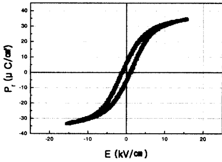
a) 10 layer stacking(5×5 mm 2 )
