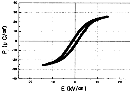
b) 10 layer stacking(10×10 mm 2 )
