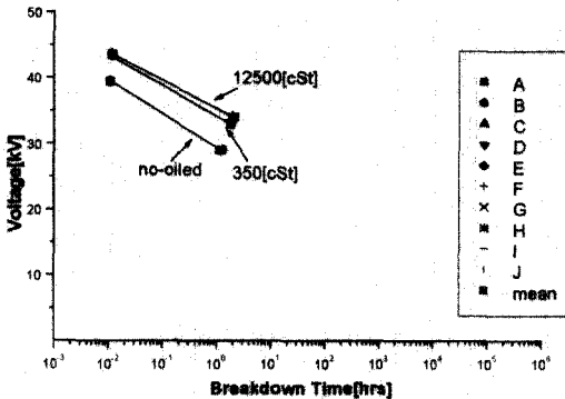
그림 4. 터폰드 에폭시와 실리콘고무 계면의 V-t 특성.
