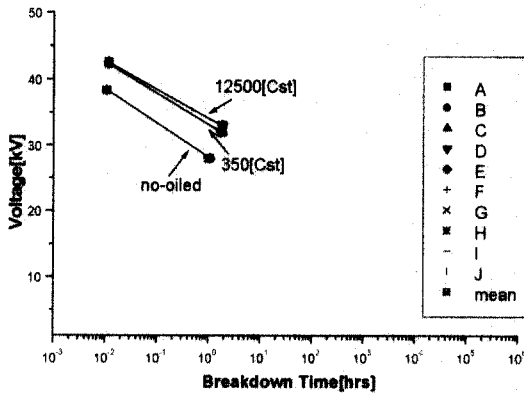
그림 5. 터프드 에폭시와 EPDM 계면의 V-t 특성. Fig. 5. V-t Characteristic of the interface between toughened epoxy and EPDM.
