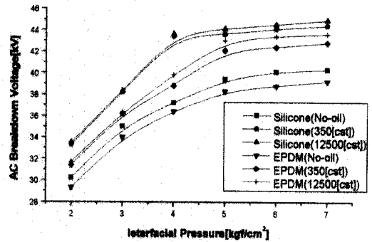
그림 3. 계면압 변화에 따른 교류 계면 파괴 전압의 변화.
