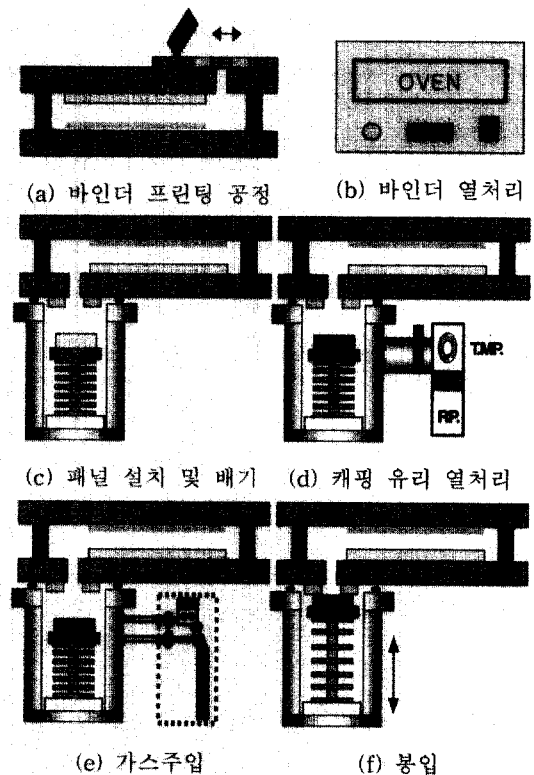
그림 2. 유기물 binder를 이용한 PDP 패키징 제작 공정 개략도.
