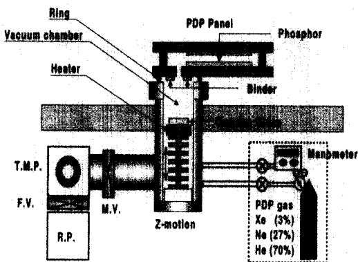
그림 1. PDP 패키징 장비 개략도.
