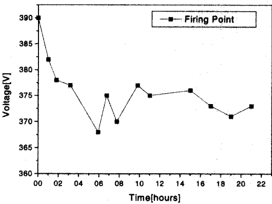
그림 6. 패널을 봉입한 후에 측정한 구동전압.
