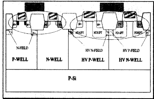
그림 1. 이중 게이트 CMOS 소자의 단면도.
