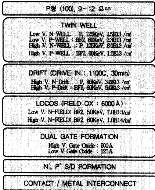
그림 2. 이중 게이트 CMOS 소자의 공정 흐름도.
