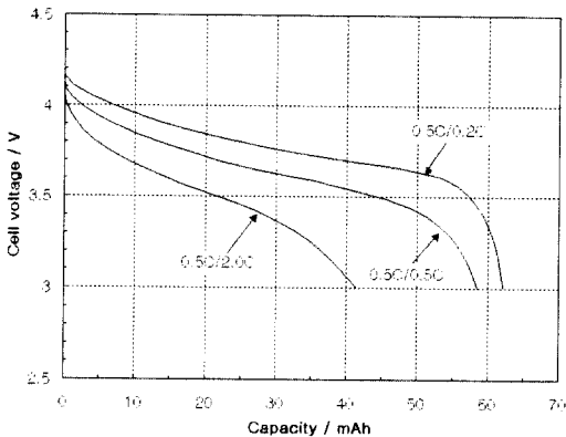
그림 7. LiCoO 2 /GPE/MCF cell의 방전율에 따른 방전곡선.
