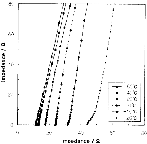
그림 2. SS/GPE/SS cell의 AC 인피던스 스펙트라. Fig. 2. AC impedance spectra of SS/GPE/SS cell with gel polymer electrolyte.
