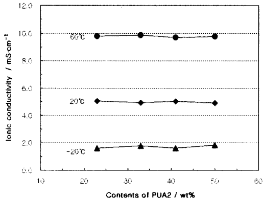
그림 5. PUA2의 함량과 이온전도도와의 관계(20°C). Fig. 5. Relationship between the ionic conductivity and the contents of PUA2.
