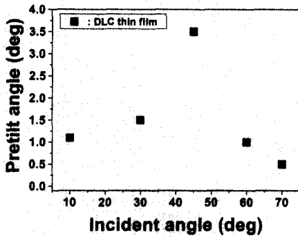
그림 4. DLC 박막 표면에 편광된 IB을 1분간 조사시의 입사각도에 따른 네마틱액정의 프리틸트각의 발생.
