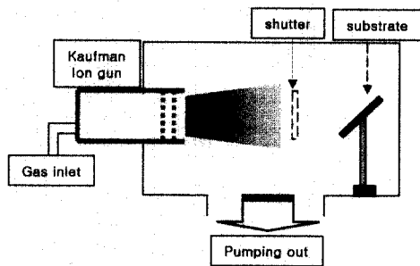
그림 1. IB 조사 시스템. Fig. 1. IB exposure system.
