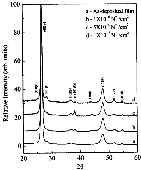
그림 2. N + 이온 주입 양에 따른 CdS 박막의 X-선 회절 패턴.
