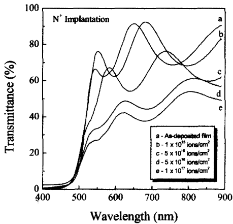
그림 4. N + 이온 주입 양을 달리하여 제조한 CdS 박막의 광 투과율. Fig. 4. Optical transmittance spectra of N + implanted CdS films with different doses.
