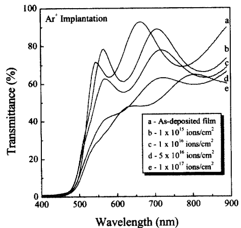
그림 3. Ar + 이온 주입 양을 달리하여 제조한 CdS 박막의 광 투과율.
