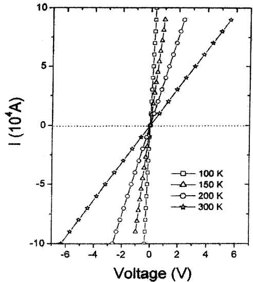
그림 1. 여러 온도에서 측정된 AlGaN/GaN 시편 (M-9)상의 In 접촉의 I-V 특성.
