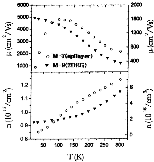
그림 2. MOVPE에 의해 성장된 AlGaIn/GaN 이종 접합(▼)과 GaN 에피층(○)의 온도의존적인 Hall 효과 측정결과.
