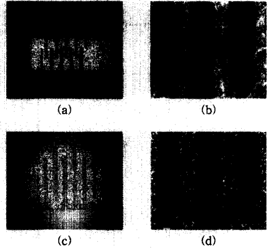
그림 5. (a), (b) 1064nm & (c), (d) 355nm 레이저를 이용한 저항체 가공 사진. Fig. 5. Photographs of resistor trimmed by (a), (b) 1064nm & (c), (d)355nm laser.
