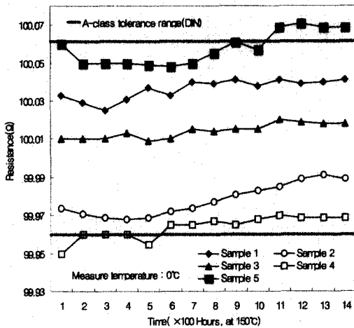
그림 8. 150°C에서 장기 신뢰성 실험. Fig. 8. Test of long terms stability at 150°C.
