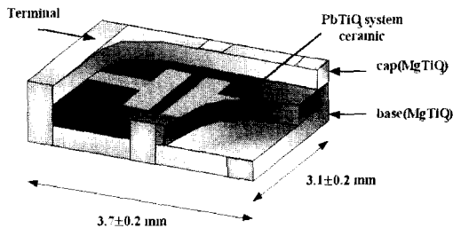
그림 1. SMD형 세라믹 필터의 내부구조.
