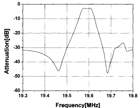
그림 2. 단독 필터의 전송특성.
