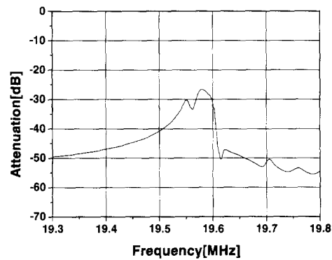
(d) C=300[pF]
