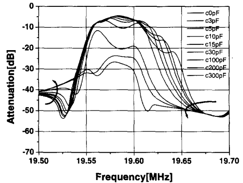
그림 5. 결합 캐패시턴스 변화에 따른 중속 연결된 필터의 좁은 범위에서의 전송특성.
