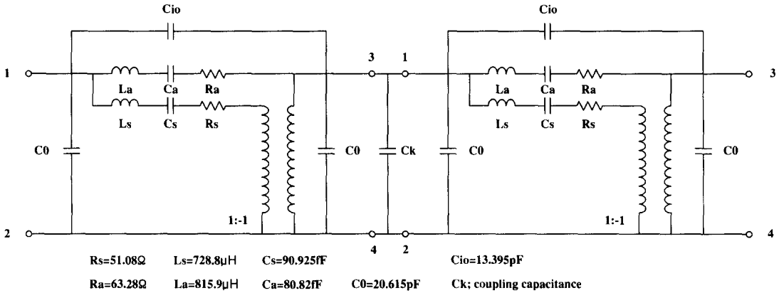
그림 3. 2개로 중속 연결된 필터의 등가회로. Fig. 3. Equivalent circuit of cascaded filter with two ones.
