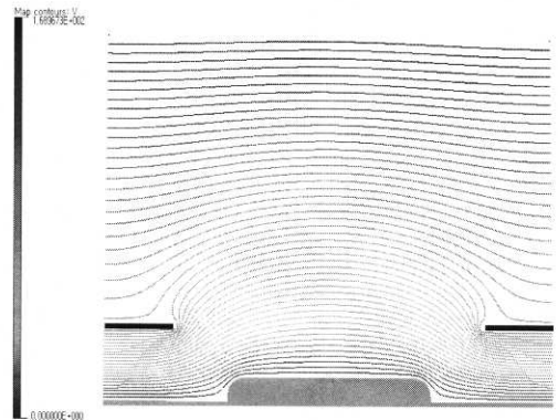
그림 2. V_g = 82 \text{ V} 인 경우 양쪽 가장자리 띠에미터의 전위 분포.
