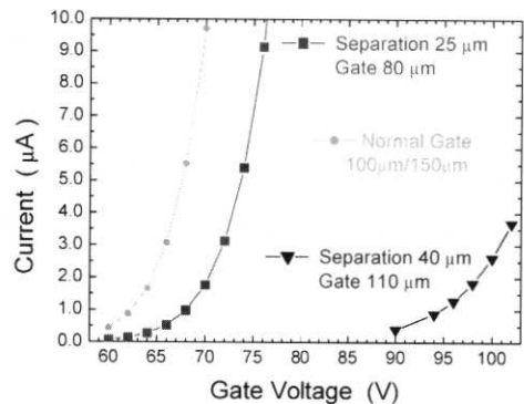
그림 7. 한쪽 가장자리 띠에미터의 전류-전압곡선. 전류는 에미터에서 방출되는 총전류를 나타낸 것이다. (▼) : 에미터-게이트 간격/게이트 구멍 폭 = 40\ \mu\text{m}/110\ \mu\text{m} , (■) : 에미터-게이트 간격/게이트 구멍폭 = 25\ \mu\text{m}/80\ \mu\text{m} , (●)는 비교를 위하여 계산한 직경 100\ \mu\text{m} 의 원형 CNT 에미터와 직경 150\ \mu\text{m} 의 원형 게이트 구멍을 가지는 삼극 구조의 전류-전압 특성이다.
