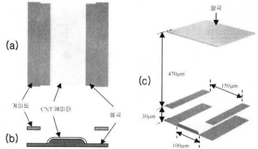
그림 1. 양쪽 가장자리 띠에미터의 구조 (a) 정면도, (b) 측면도, (c) 계산에 이용된 수치들.
