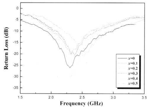
그림 9. Mo이 치환된 \text{BiNbO}_4 세라믹 모노폴 안테나의 반사손실 측정 결과.
