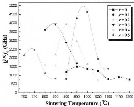
그림 7. 소결온도에 따른 \text{Bi}(\text{Nb}_{1-6x/5}\text{Mo}_x)\text{O}_4 + 0.1\text{wt.}\% \text{CuO} 세라믹스의 품질계수 변화.
