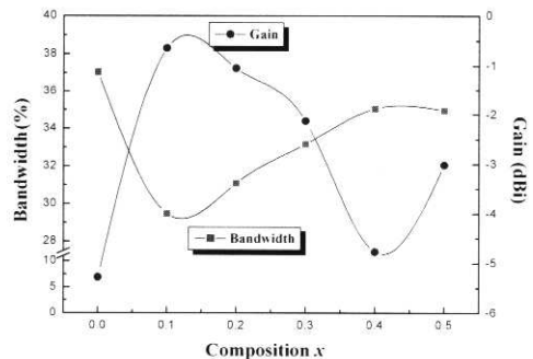
그림 10. Mo의 치환량에 따른 \text{Bi}(\text{Nb}_{1-6x/5}\text{Mo}_x)\text{O}_4 + 0.1\text{wt.}\% \text{CuO} 세라믹 모노폴 안테나의 임피던스 대역폭과 이득 변화.
