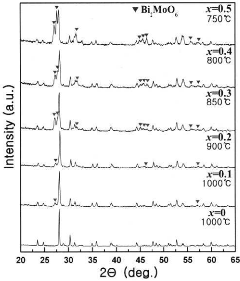
그림 3. 소결밀도가 최대에 이르는 온도에서 소결한 Bi(Nb 1-6x/5 Mo x )O 4 + 0.1wt.%CuO세라믹스의 XRD 패턴.
