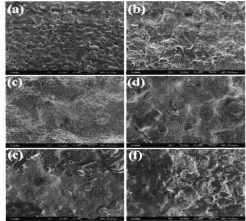
그림 4. 조성별 적정 온도에서 소결한 Bi(Nb 1-6x/5 Mo x )O 4 + 0.1wt.%CuO 세라믹스의 FE-SEM 사진.
