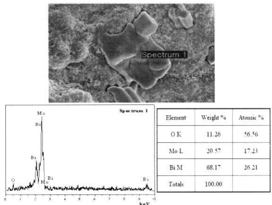
그림 5. 850 °C에서 소결한 30at.% Mo이 치환된 Bi(Nb 1-6x/5 Mo x )O 4 + 0.1wt.% CuO 세라믹스의 EDS 스펙트럼.
