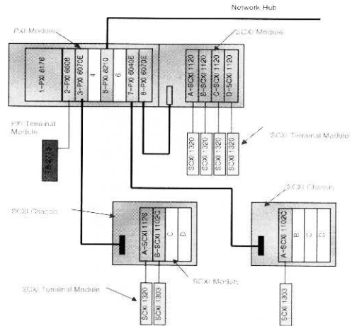
그림 3. 계측시스템의 모듈 구성. Fig. 3. Module composition of measurement system.
