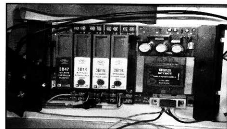
그림 5. 3B Module 외형. Fig. 5. Shape of 3B Module.
