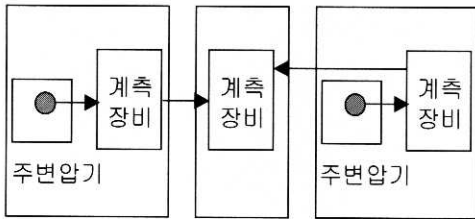
그림 1. 주변압기 온도측정 구성도. Fig. 1. Composition of temperature measurement for main transformer.
