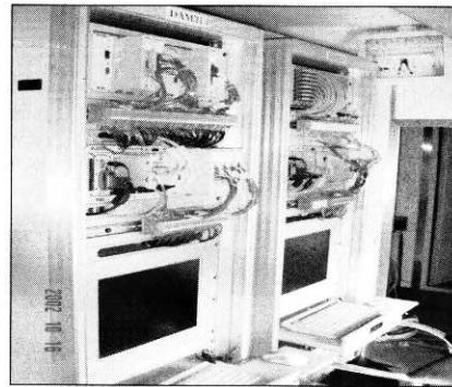
그림 4. 계측시스템의 외형도. Fig. 4. Shape of measurement system.
