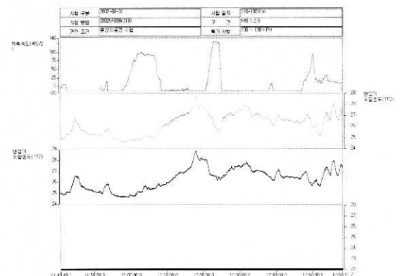
그림 14. 140km/h에서의 변압기 온도특성 변화. Fig. 14. Main Transformer temperature characteristics in 140km/h.
