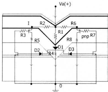
그림 2. 직류 등가회로 모델. Fig. 2. DC equivalent circuit.
