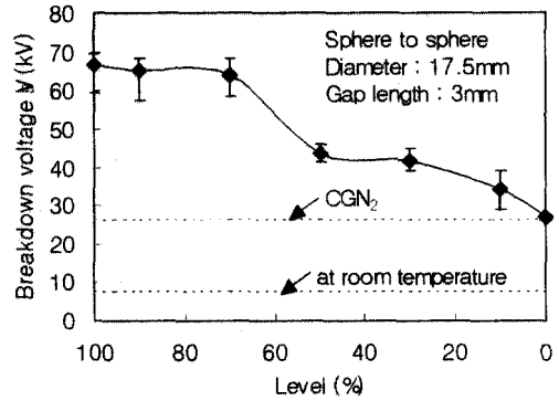
그림 10. LN₂와 CGN₂의 복합계에서 LN₂의 레벨에 따른 절연파괴전압. Fig. 10. V B of complex condition of CGN 2 above a LN 2 as function of LN 2 level.
