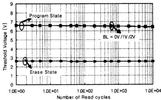
그림 6. 읽기 반복 회수에 따른 SONOS 플래시 어레이의 읽기 간섭특성.
