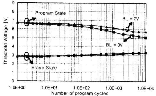
그림 4. 프로그램 반복 회수에 따른 SONOS 플래시 어레이의 게이트 간섭특성: cell(C).
