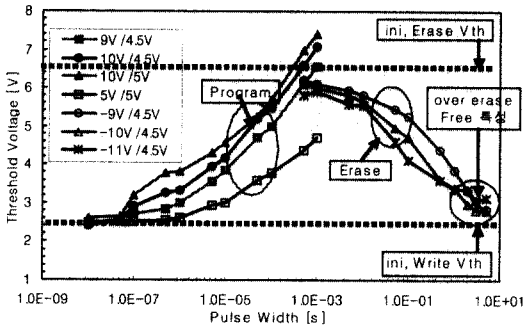
그림 3. SONOS 플래시 메모리 어레이에서 선택된 셀의 스위칭 특성 (채널 W/L=0.6\mu\text{m}/0.4\mu\text{m} ).
