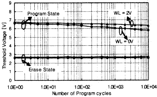
그림 5. 프로그램 반복 회수에 따른 SONOS 플래시 어레이의 드레인 간섭특성: cell(B).
