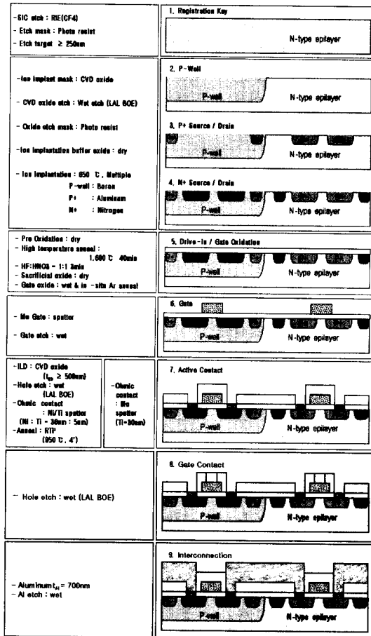
그림 1. 전체 SiC CMOS 공정 순서도. Fig. 1. Overall process flow of SiC CMOS.
