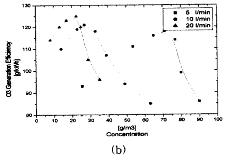
그림 10. 가스 유량과 소비 전력에 따른 오존 발생 특성. 가스 압력 : 1.2 atm, 방전 거리 : 0.8 mm.
