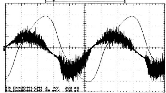
그림 2. 전원의 전압, 전류 파형.
