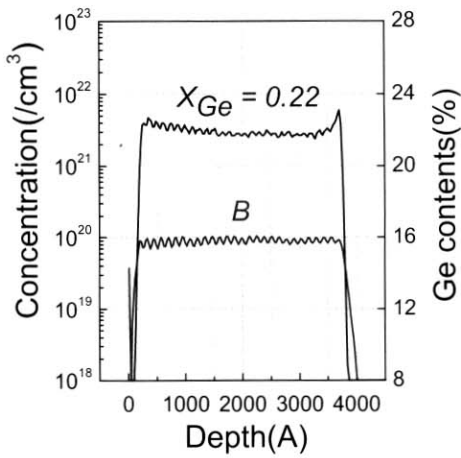
그림 6. 증착과 식각의 반복공정을 실시한 시편의 SIMS 분석 결과.
