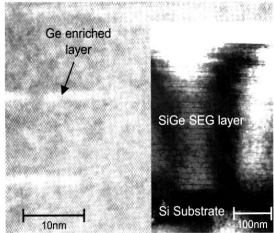
그림 7. 고배율의 단면 TEM 분석 사진.
