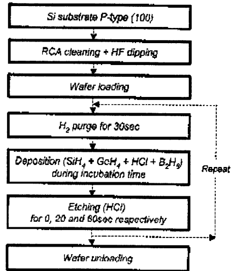
그림 1. 선택적 실리콘-게르마늄 단결정 성장법의 공정 순서도.
