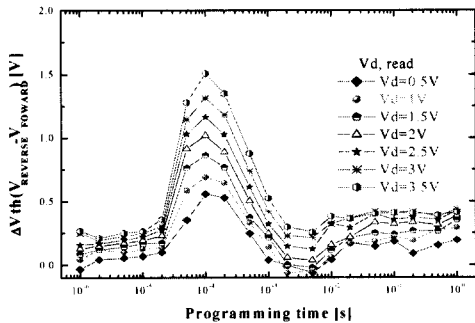
그림 5. 읽기 전압변화에 따른 멀티 비트 프로그래밍 특성.
