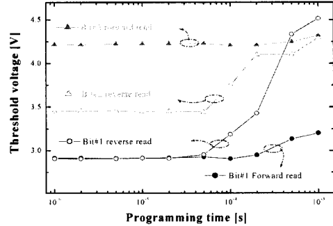
그림 6. 멀티 비트의 프로그램 특성.
