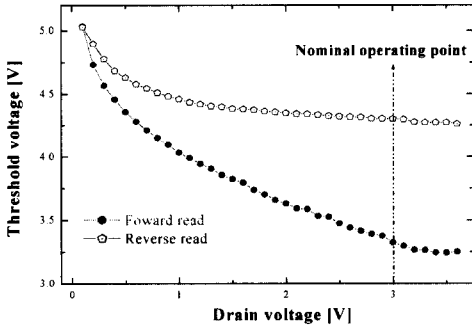
그림 4. 멀티비트의 문턱전압 대 읽기 동작을 위한 드레인전압.
