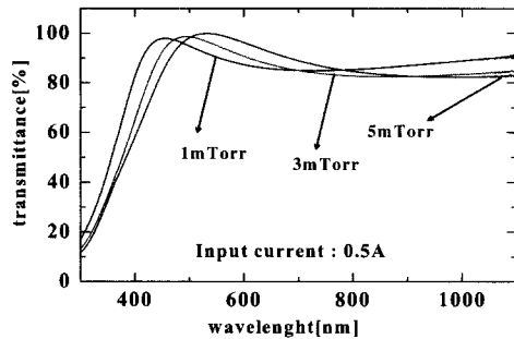
그림 6. 제작되어진 ITO 박막의 광투과율.
