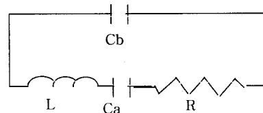
그림 6. 그림 3의 설계로 제작된 혼으로부터 얻은 등가회로.
