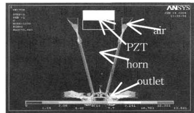
그림 5. 초음파 혼의 냉각구조. Fig. 5. Cooling mechanism for ultrasonic horn.
